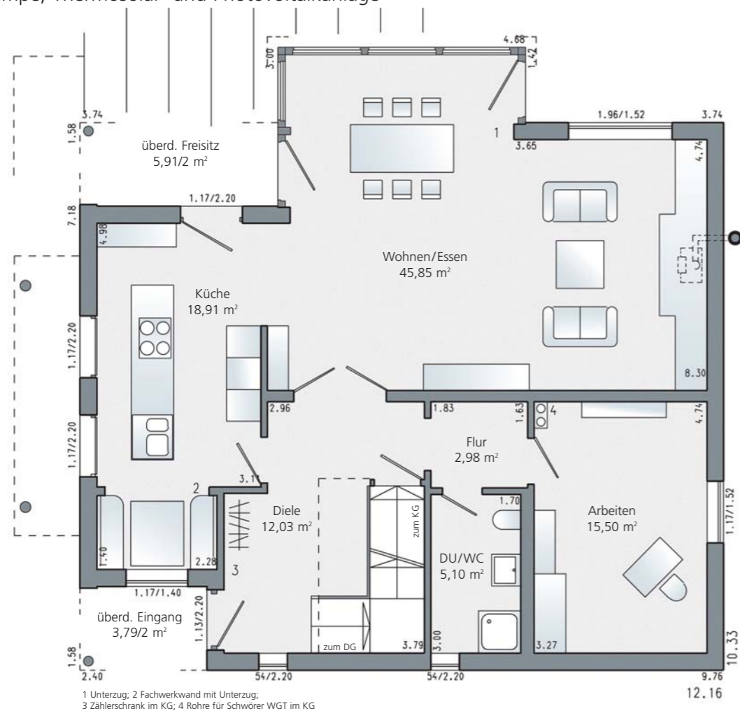
Erdgeschoss Plan 481.1 105,22 m² Wohnfläche Maßstab 1:100
