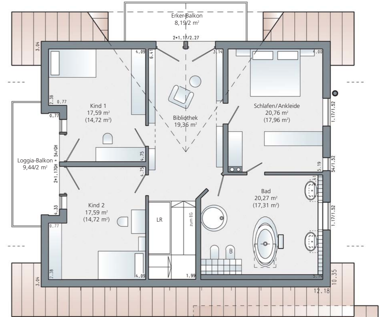
Dachgeschoss Plan 481.1 DN 35°, KN 105 cm 104,39 m² nutzbare Grundfläche 92,89 m² Wohnfläche Maßstab 1:100
